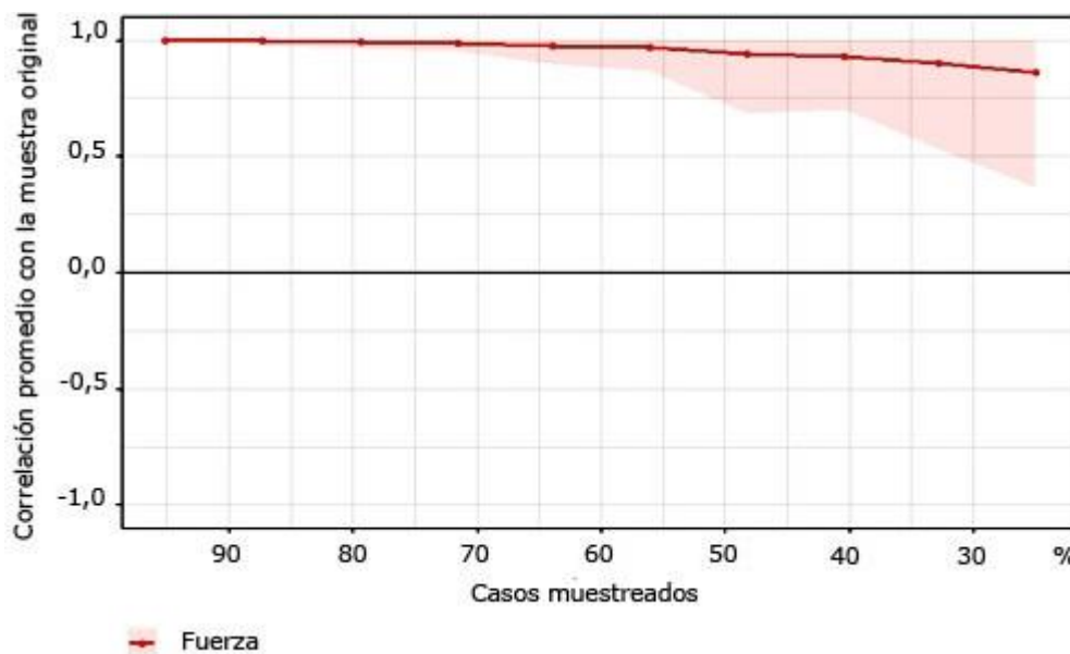
Fig. 3 – Estabilidad del índice de centralidad de fuerza.
